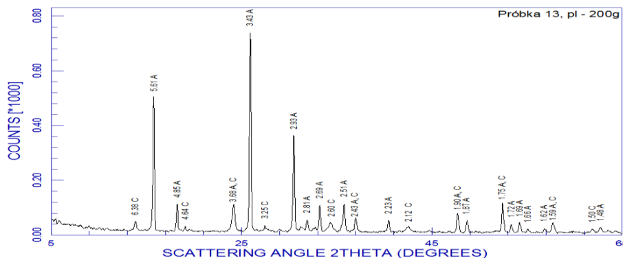
Rys. 1. Dyfraktogram materiału zeolitowego (próbka 13).
