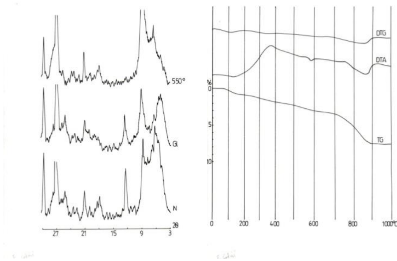
Rys. 3. Dyfraktogram i dewarytogram gleby rozwijającej się z gruntów pogórnich-analiza całej próbki bez rozfrakcjonowana Fig. 3. x-ray diffractogram and derivatogram of soil developing from post mining grounds of a whole sample
