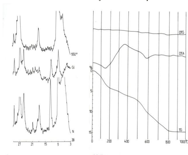
Rys. 2. Dyfraktogram i dewarytogram świeżego gruntu pogórnicznego – analiza frakcji < 0,002\text{mm}
