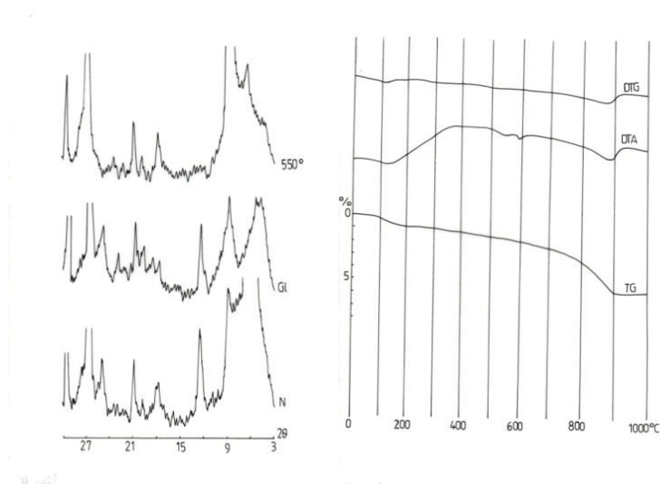
Rys. 1. Dyfraktogram i dewarytogram świeżego gruntu pogórnicznego – analiza całej próbki bez rozfrakcjonowania
