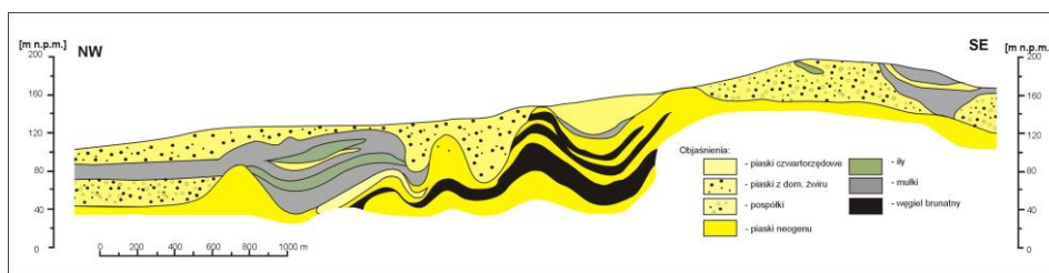
Rys. 7. Schemat budowy geologicznej złoża Zielona Góra Fig. 7. Geological structure scheme of the deposit Zielona Góra
