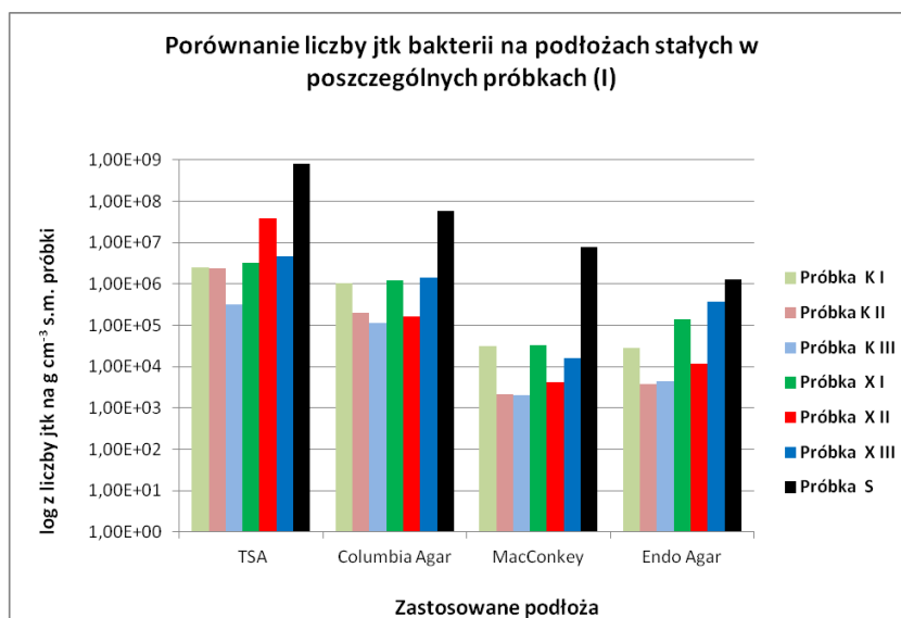
Rys. 1. Liczebność jtk bakterii na czterech podstawowych, stosowanych w badaniach ilościowych podłożach stałych Fig. 1. Number of CFU of bacteria on the four used in quantitative research, primary solid medium
