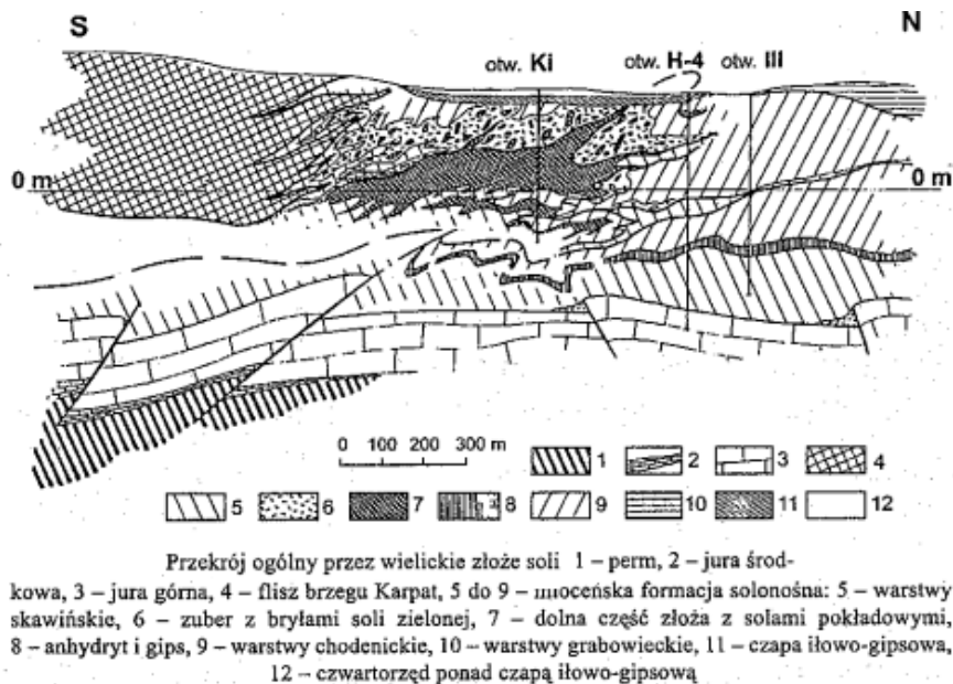
Rys. 1. Przekrój geologiczny przez złoża soli w Wieliczce [Poborski, 1965] Fig. 1. Geological cross-section in the Wieliczka salt deposits [Poborski, 1965]
